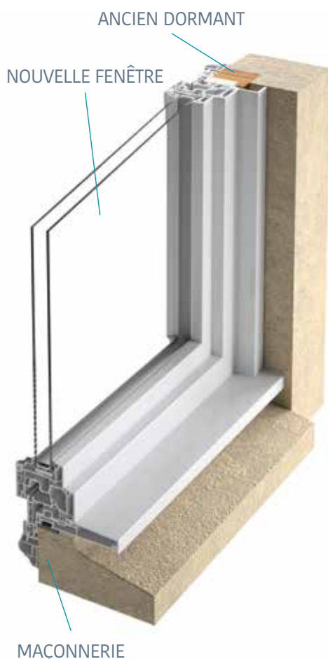
Pose en rénovation avec dépose de l'appui bois
